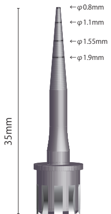
インプラントリムーバー：ロング
